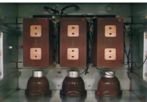
支柱式
